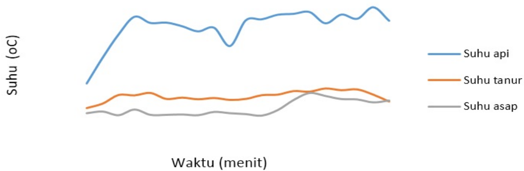
Gambar 2. Fluktuasi suhu selama berlangsungnya proses pirolisis TKKS untuk menghasilkan arang hayati TKKS dan asap cair.
